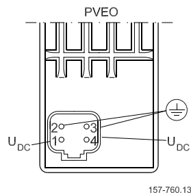
Deutsch® version of PVEO
