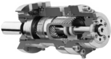
Rotary Aktüatör Kesiti
